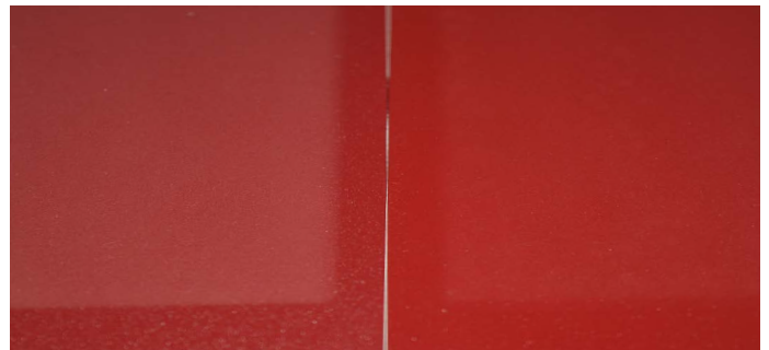
Retención de color: envejecimiento acelerado QUVB 600h Alesta® AP izquierda/Alesta® SD derecha
